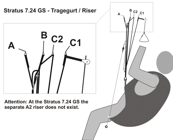
Bild 3: Aufbau Tragegurt Stratus 7.24 GS
