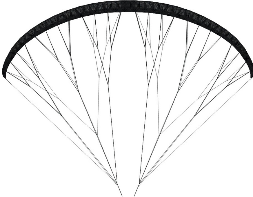
Bild 1: Gittermodell Stratus 7 GS (Frontansicht)
