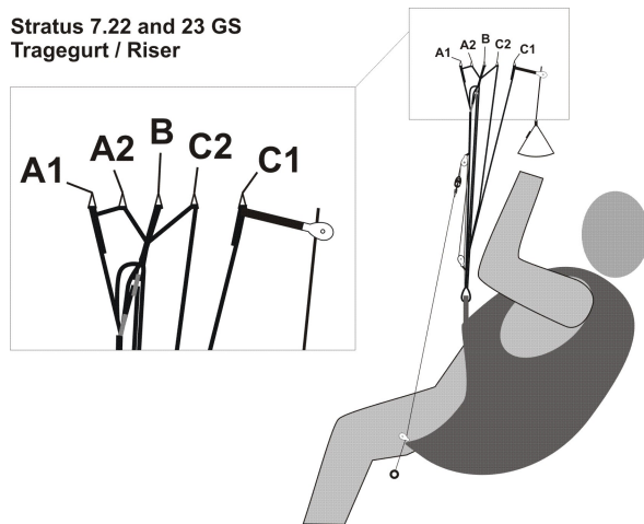
Bild 2: Aufbau Tragegurt Stratus 7.22 und 7.23 GS
